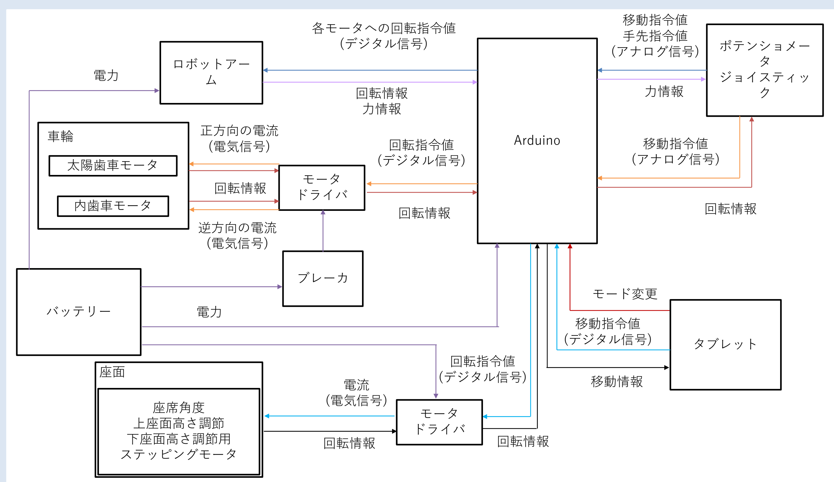
図6：システム構成図
