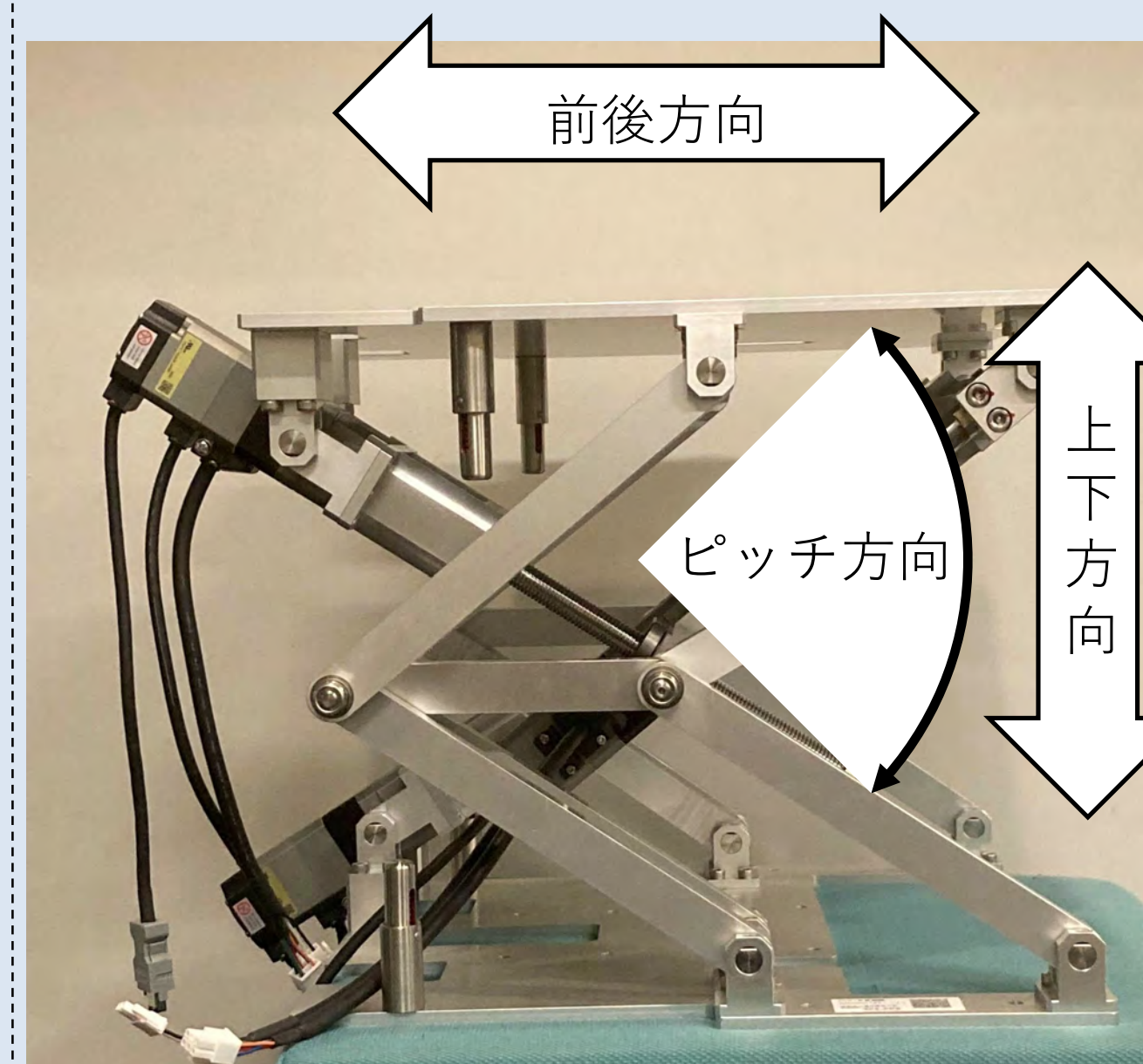
図9：座面部の動作
