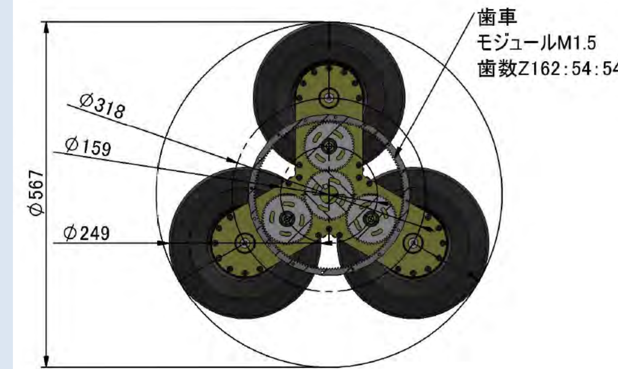
図8：遊星歯車の図面
