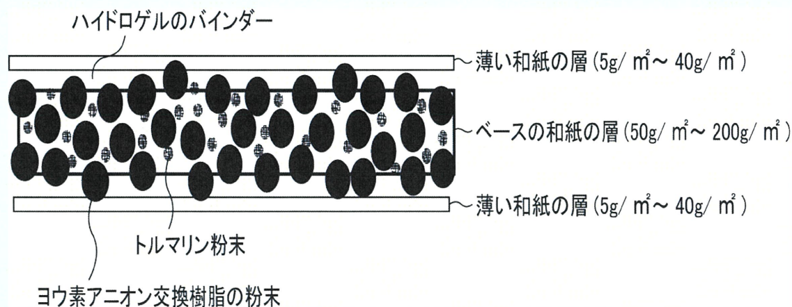
高機能性消臭和紙の実施形態断面図
