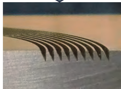
加工断面形状 (被切削材: NAK55)
