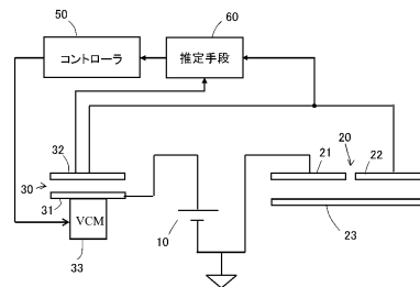
実施形態に係る静電浮上装置
